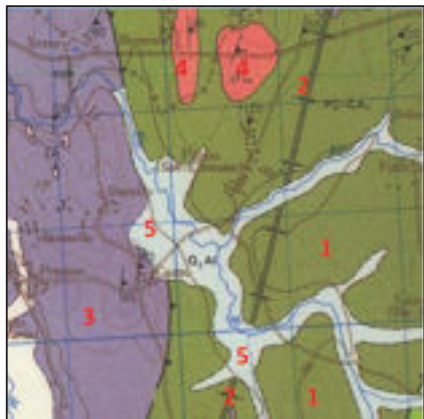
Composición xeolóxica da parroquia.
