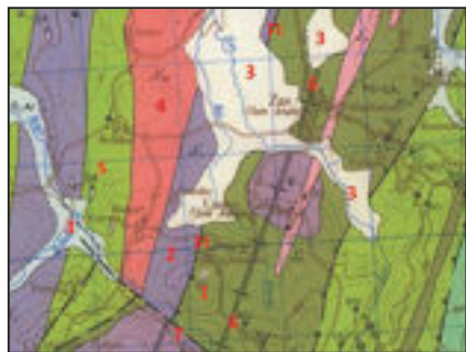
Composición xeolóxica da parroquia ( http://info.igme.es/cartografiadigital/datos/magna50/jpgs/d0_G50/Editado_MAGNA50_68.jpg )
