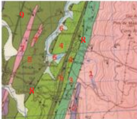
Composición xeolóxica da parroquia: http://info.igme.es/cartografiadigital/datos/magna50/jpgs/d0_G50/Editado_MAGNA50_68.jpg
