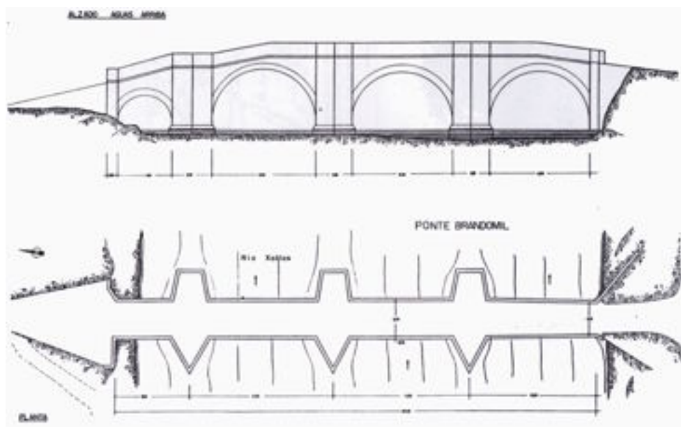
Alzado e planta da Ponte Vella de Brandomil (S. Alvarado e outros 1989)
