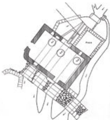
Planta do muíño do baruto do Allo (Roberto Mouzo, 1994)
